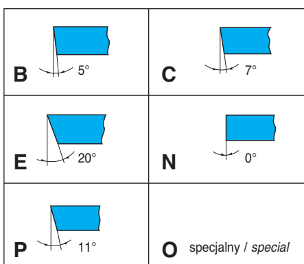
Kąt przyłożenia \alpha_n 4 Normal clearance angle
